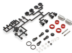
FAW302 FZアルミダンパーセット (FZ02/O2L/D2) FZ Aluminum Shock Set (FZ02/O2L/D2)
