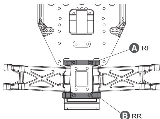
サスホルダー Sus. Holder
