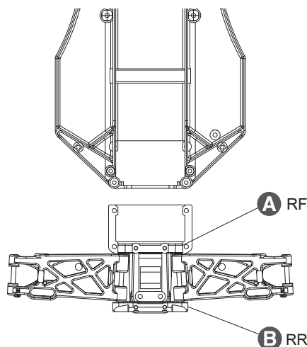
サスホルダー Sus. Holder
